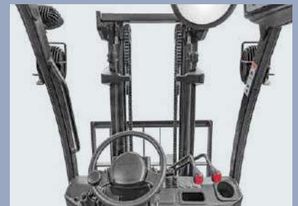
Das Weitsicht – Hubgerüst ist so orientiert, dass es die Sicht möglichst wenig behindert wird. Auch die verbreiterte Öffnung des Gabelträgers wirkt in diesem Sinn. Durch den hohen Angelpunkt des Neigungszylinders wird die Last optimal ausbalanciert, so dass sich das Hubgerüst stabil fahren lässt.
